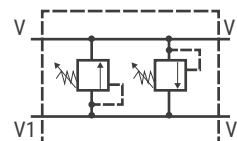
2 Schemat obwodu instalacji hyd.
