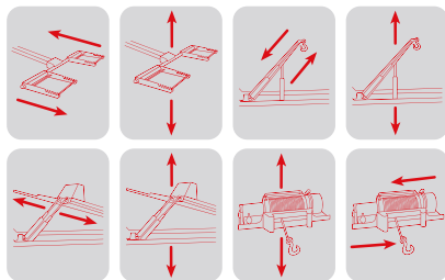
3 Zestaw symboli opisowych do rozdzielaczy
