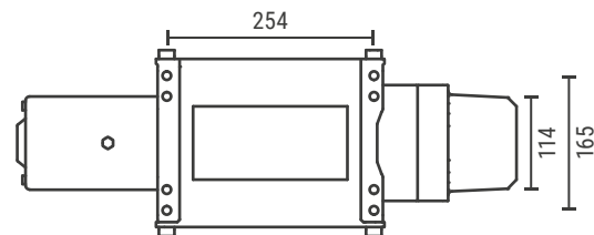
Rozstaw śrub Rhino 8/12/15
